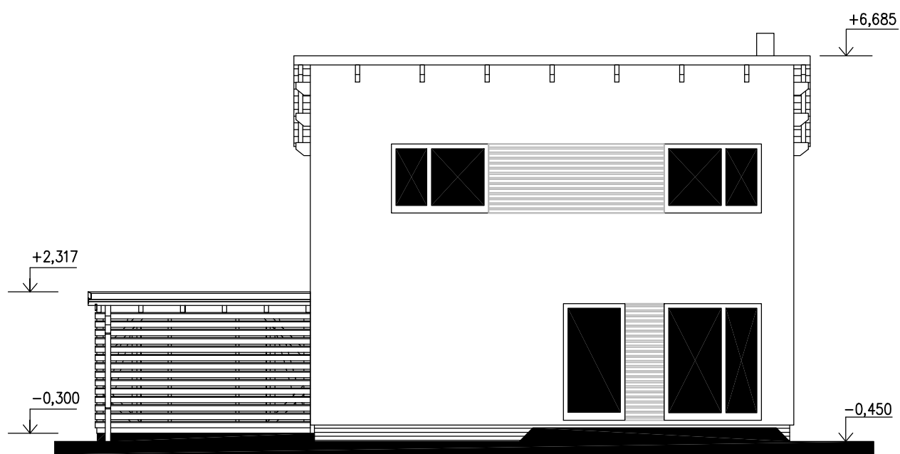
POHLED ZAHRADNÍ
